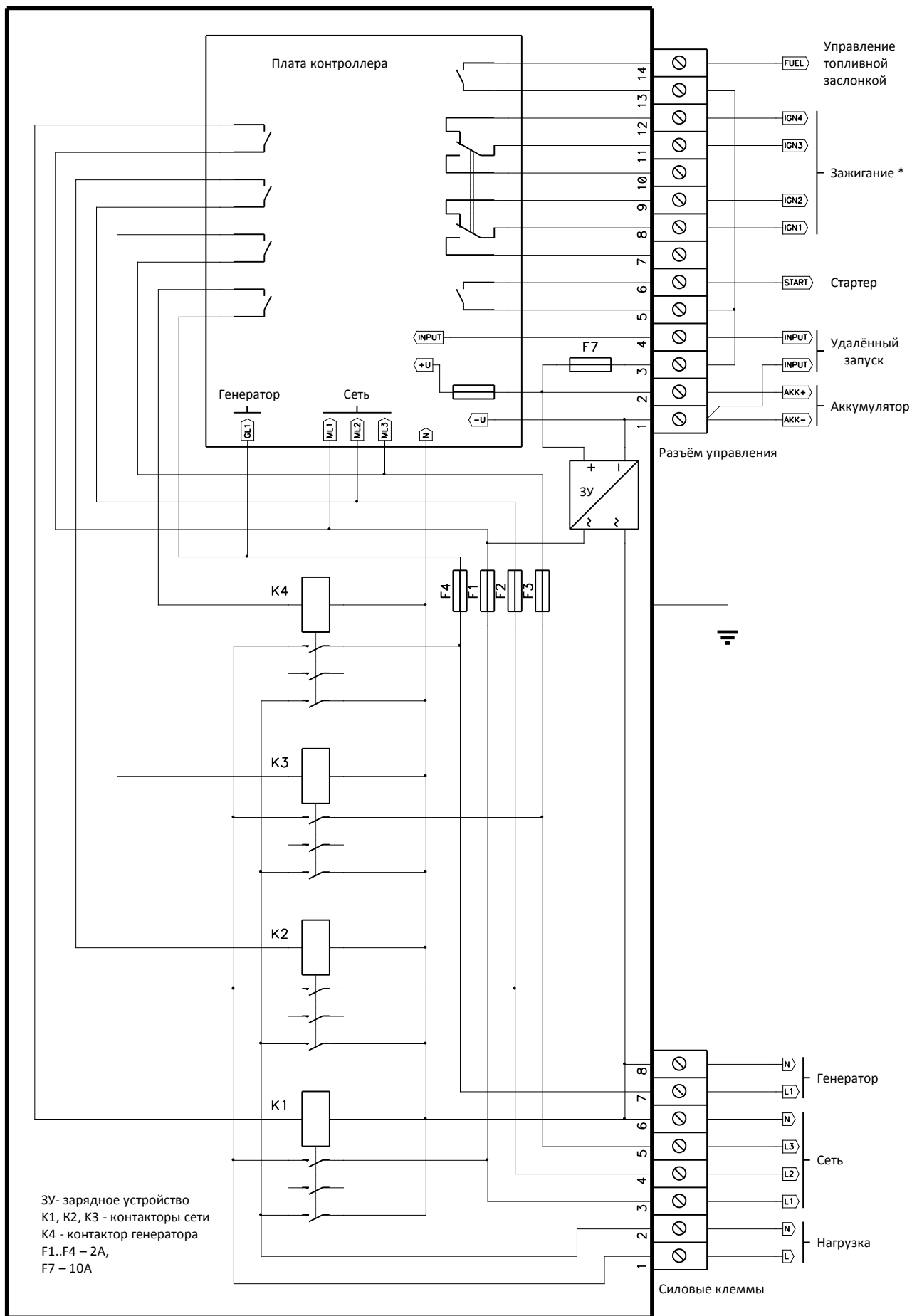
Рис 6.2. Пример схемы подключения контроллера AVR311ME / AVR311CE.
