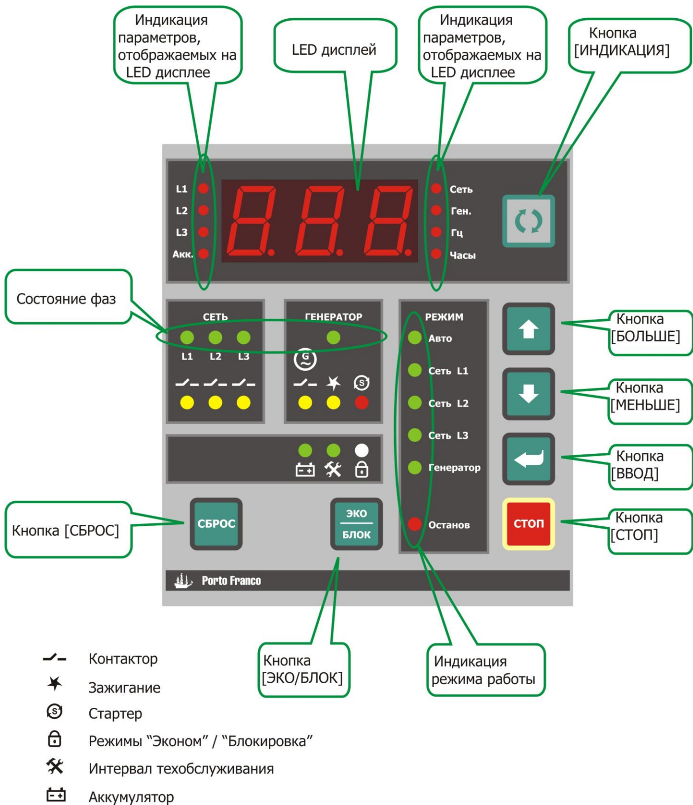
Рис. 5.2. Панель индикации и управления
