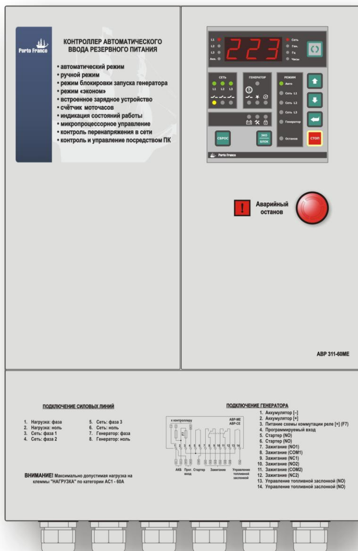
Рис. 5.1. Внешний вид контроллера АВР.
